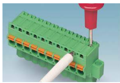
Entegre test bağlantıları
