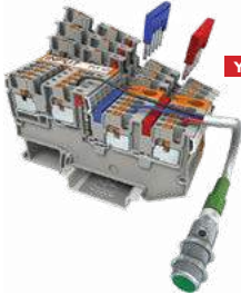
PTTB 2,5-DIO/O-U
