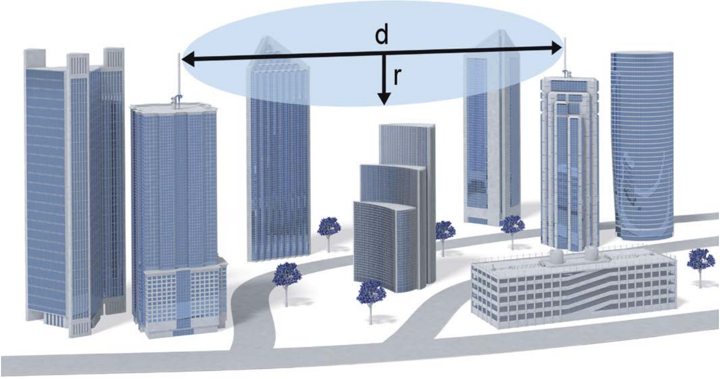
Şekil : Fresnel-Zone
