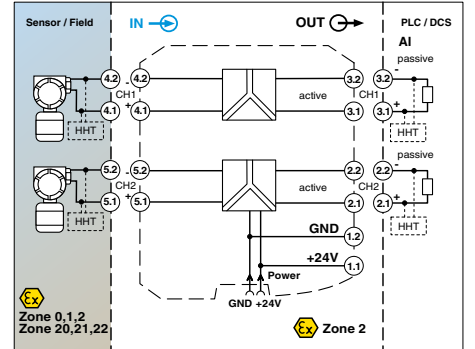
MACX MCR-EX-SL-RPSSI-2I-2I için bağlantı şekli
