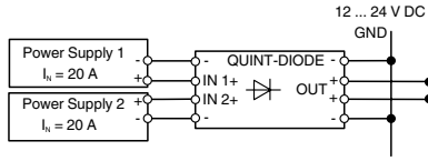
2 adet 20A güç kaynağının diyot modülüne bağlantısı
