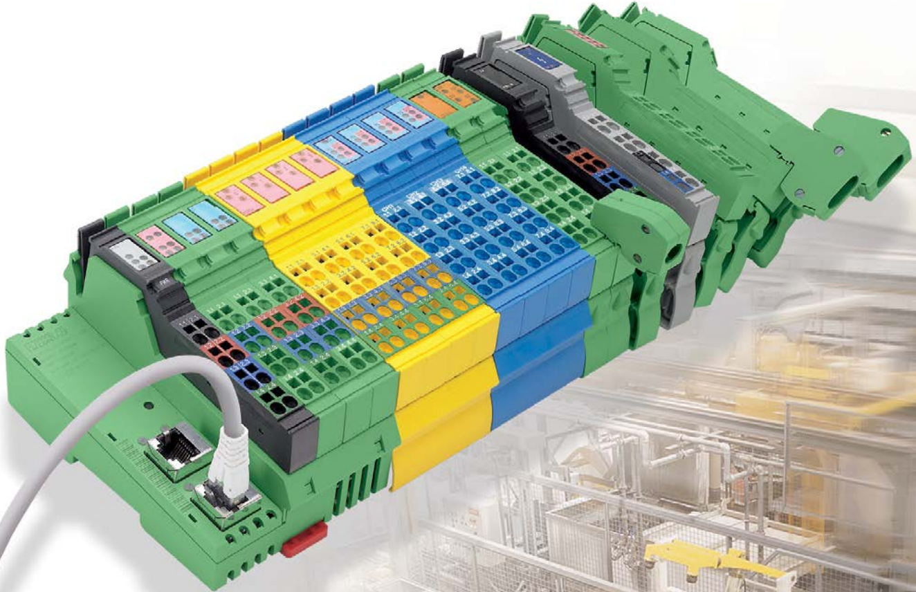
ILB ETH 24 DI16 DIO16-2TX
