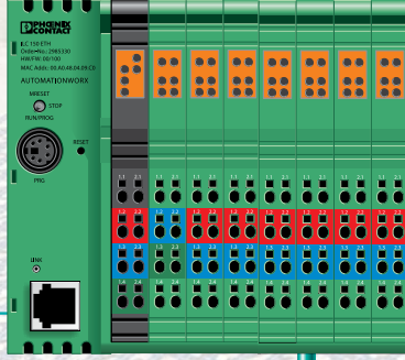
Kontrolör
