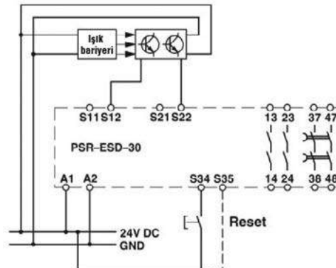
2981800 Örnek bağlantı şeması
