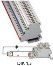
DIK 1,5
