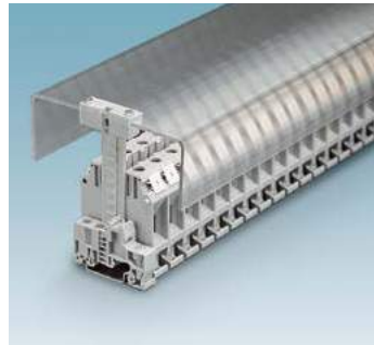
A/U profilin, yüksekliği ayarlanabilir VAH taşıyıcı ve CLIPFIX 35 durdurucu ile uygulaması
