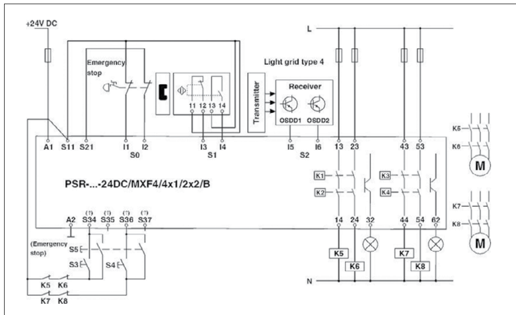
2903260 Örnek bağlantı şeması
