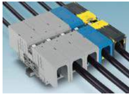
RBO 8... , HC-RBO 8... koruma kapağı ile birlikte
