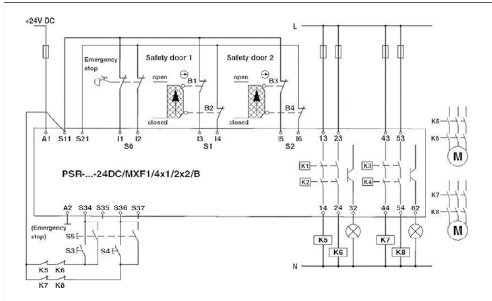
2902725 Örnek bağlantı şeması
