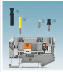
PTU 6-T-P
