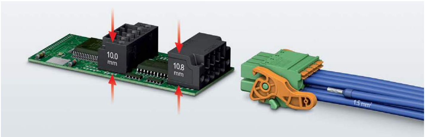
DMCV1,5/...-G1F-3,5P20THR
