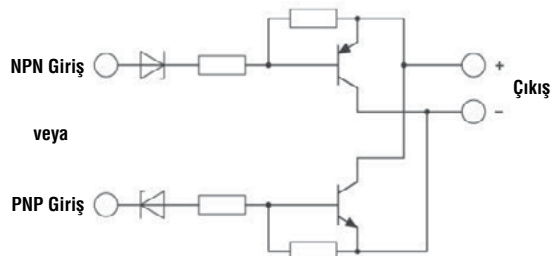
DEK-TR/INV bağlantı şekli
