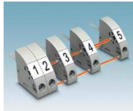
Tespit pinli tipler hazır bloklar oluşturmak için kullanılarak montaj zamanı kısaltılır
