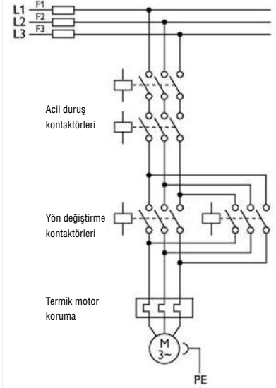
Klasik bağlantı
